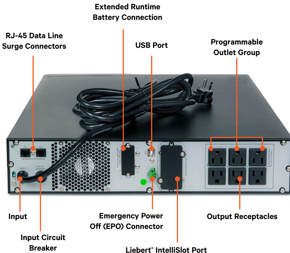
Liebert® PSI5-1500 model
