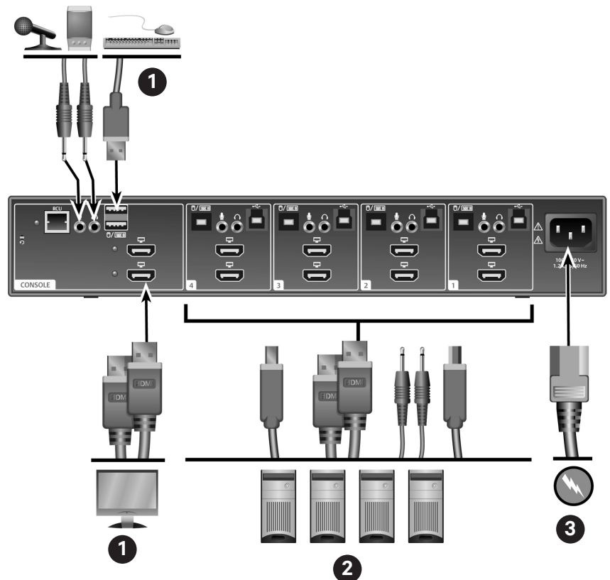
Vertiv™ Avocent® SV 340H Switch Shown
